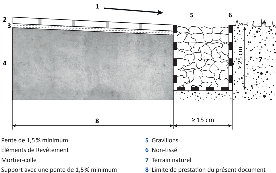
Figure 3 : sols extérieurs sur terre-plein avec terrain naturel au nu du revêtement
