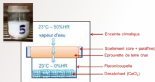
Descriptif d'un essai de perméabilité à la vapeur d'eau.
