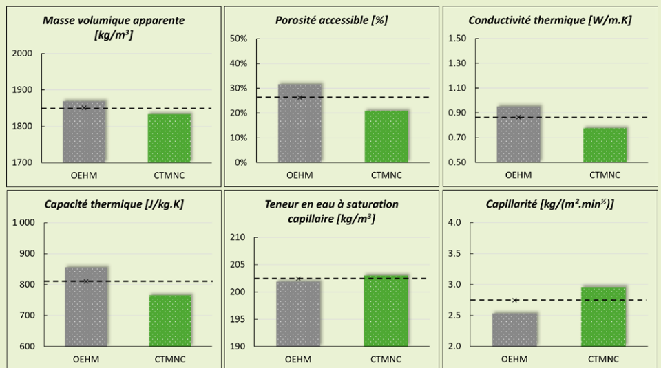
Comparaison de résultats de caractérisation, OEHM (Equipe DMS) et CTMNC, pierre de Vers-Pont-du-Gard.
