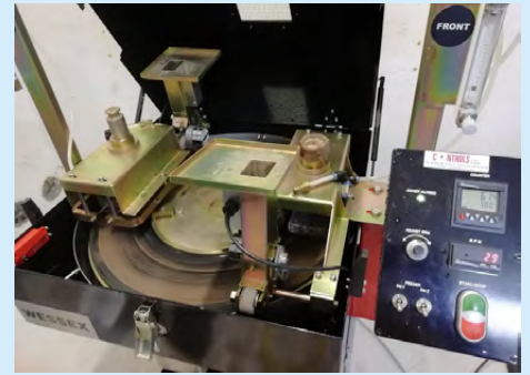
La « polish paver machine » - Photo : CTMNC
