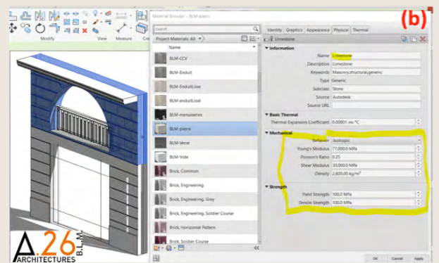
Exemple de projet BIM de construction de 150 logements à Puteaux (Architecte : A26 - Atelier BLM ; BET : Codibat) : (a) Perspectives et modélisation du projet incorporant de la pierre naturelle ; (b) Propriétés physico-mécaniques de la pierre mise en œuvre sous le logiciel de modélisation BIM (Revit)
