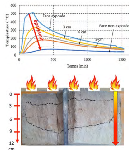
Figure 2 - Evolution du profil de température d'une pierre calcaire (12 cm d'épaisseur) au cours d'un cycle de chauffage-refroidissement (exposition unificale à une température maximale de 500 °C)
