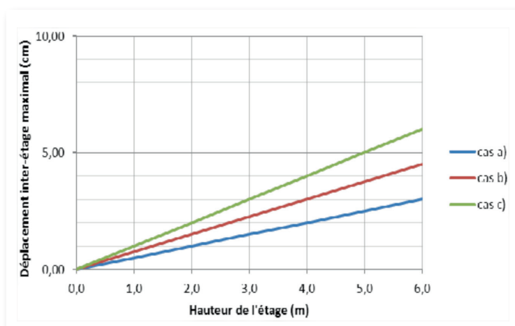
Figure 2-4: Valeurs des déplacements inter-étages maximaux sous séisme fréquent
