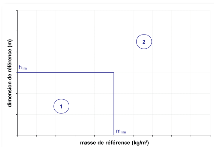
Figure 1-2: Domaine d'application pour la prise en compte de l'action sismique
